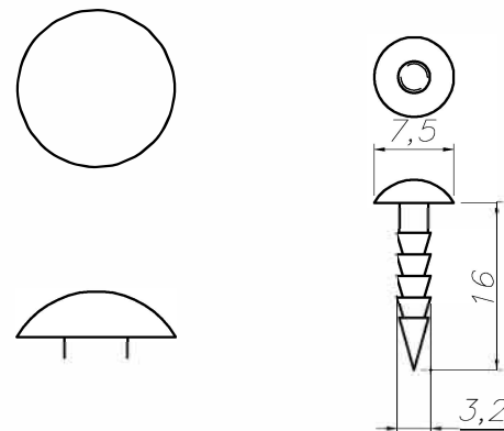
PG7,5X3,2X16R/NI
