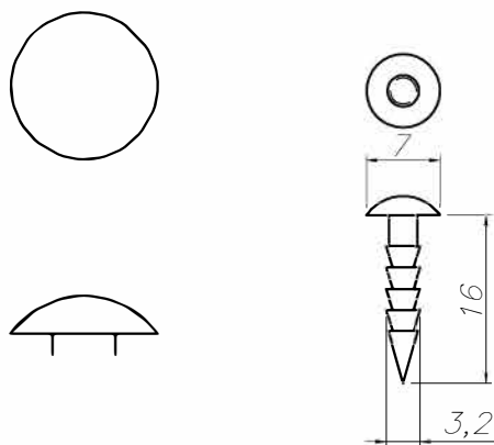
PG7X3,2X16R/NI
