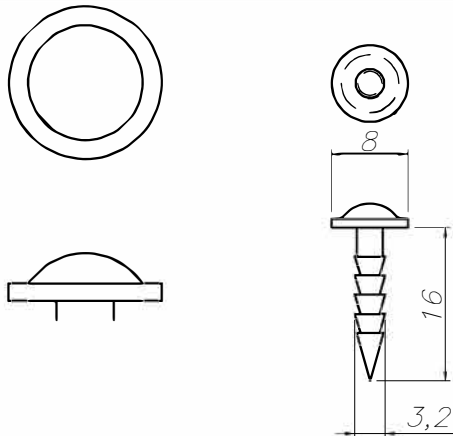
PG8X3,2X16FG/NI
