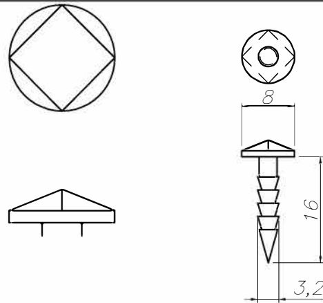
PG8X3,2X16PR/NI
